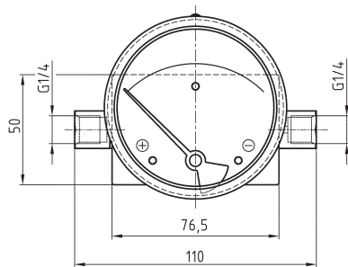
Anschluss rechts und links, seitlich
