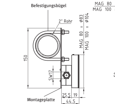
Montageplatte und Befestigungsbügel
